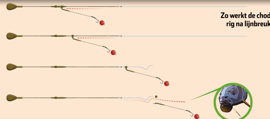
Chod rig
